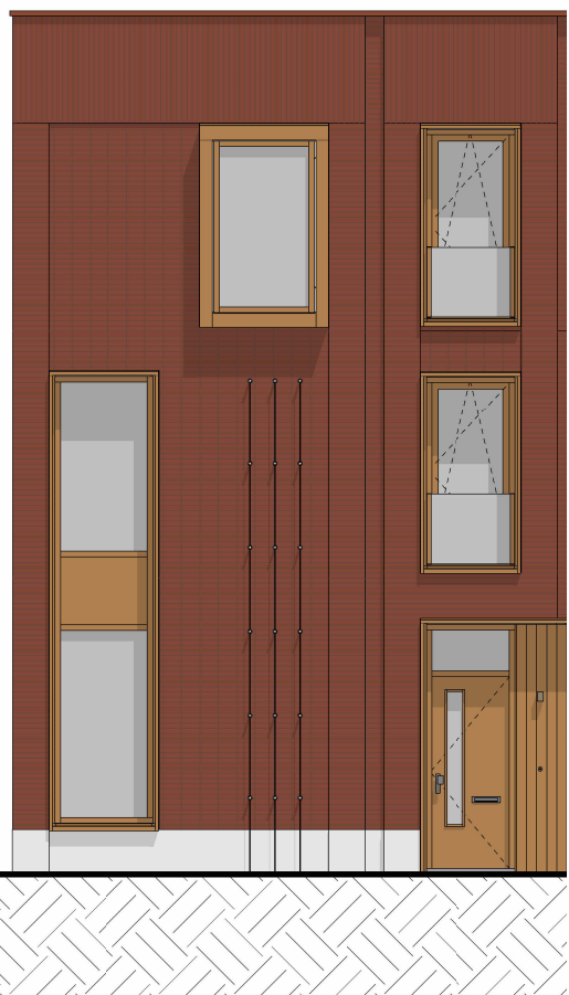
voorgevel 1 : 100
