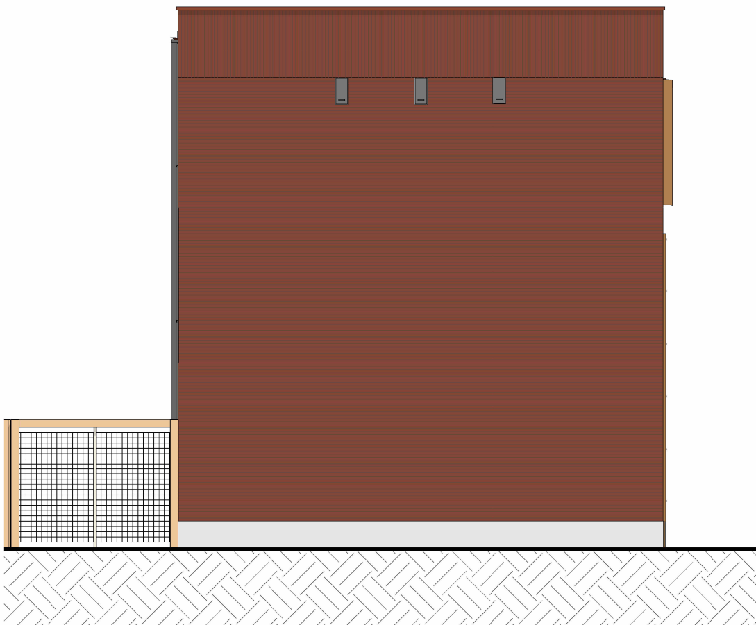
kopgevel 1 : 100
