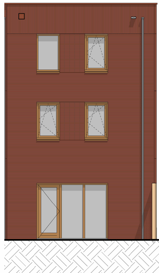
achtergevel 1 : 100
