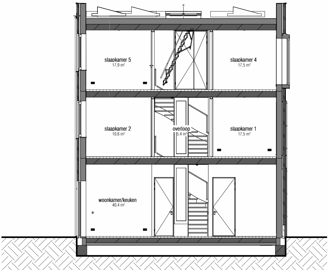
doorsnede 1 : 100
