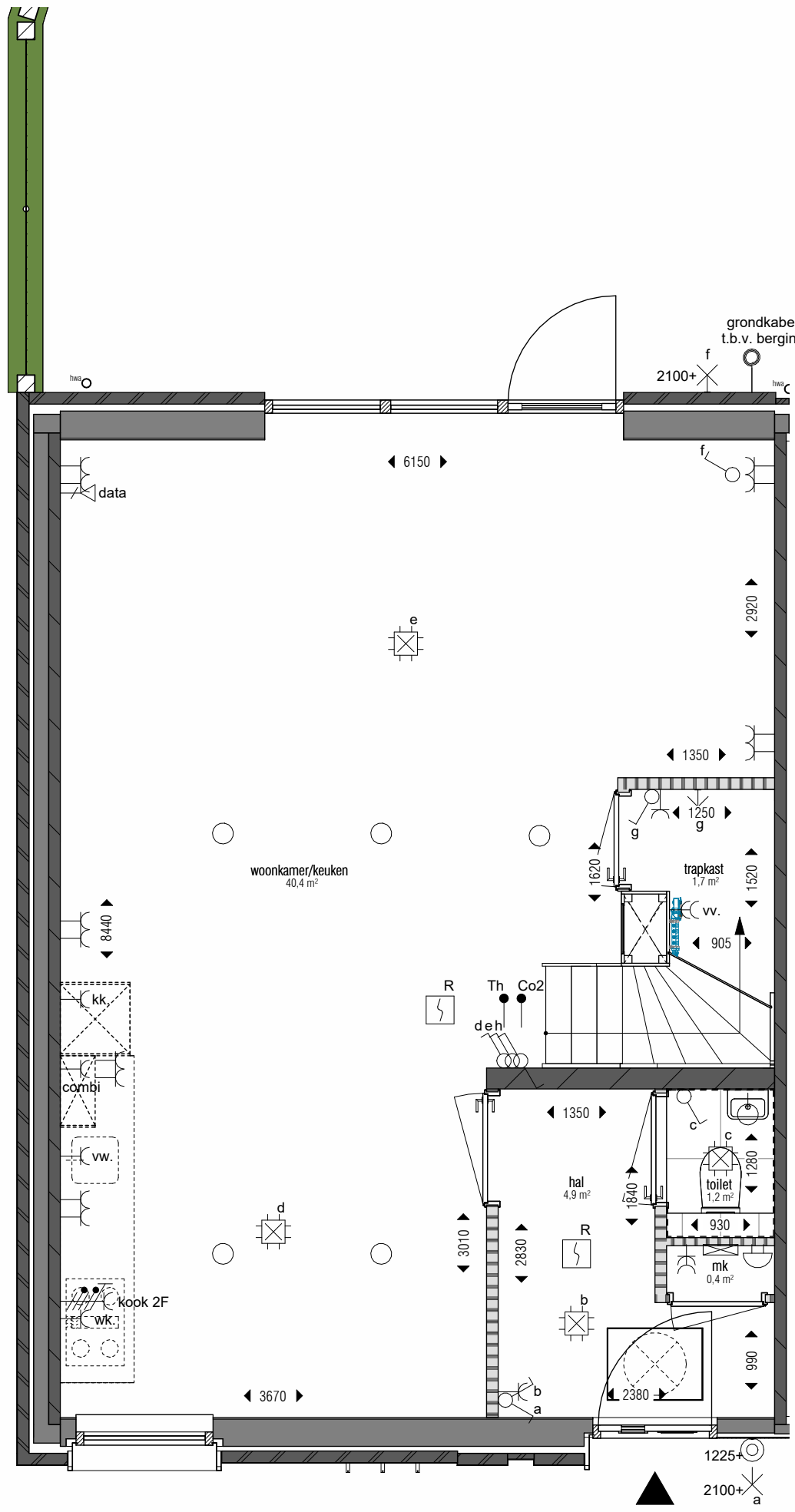
begane grond 1 : 50
